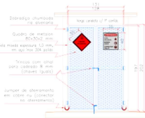
GRADIL (Frontal) ESCALA 1:25 Material: aço carbono galvanizado pintado com esmalte branco, espessura seca 120 micrômetros. Tela: tipo moeda em aço inox 304 polido, espessura 1,0 mm. Soldagem: eletrodo revestido.
